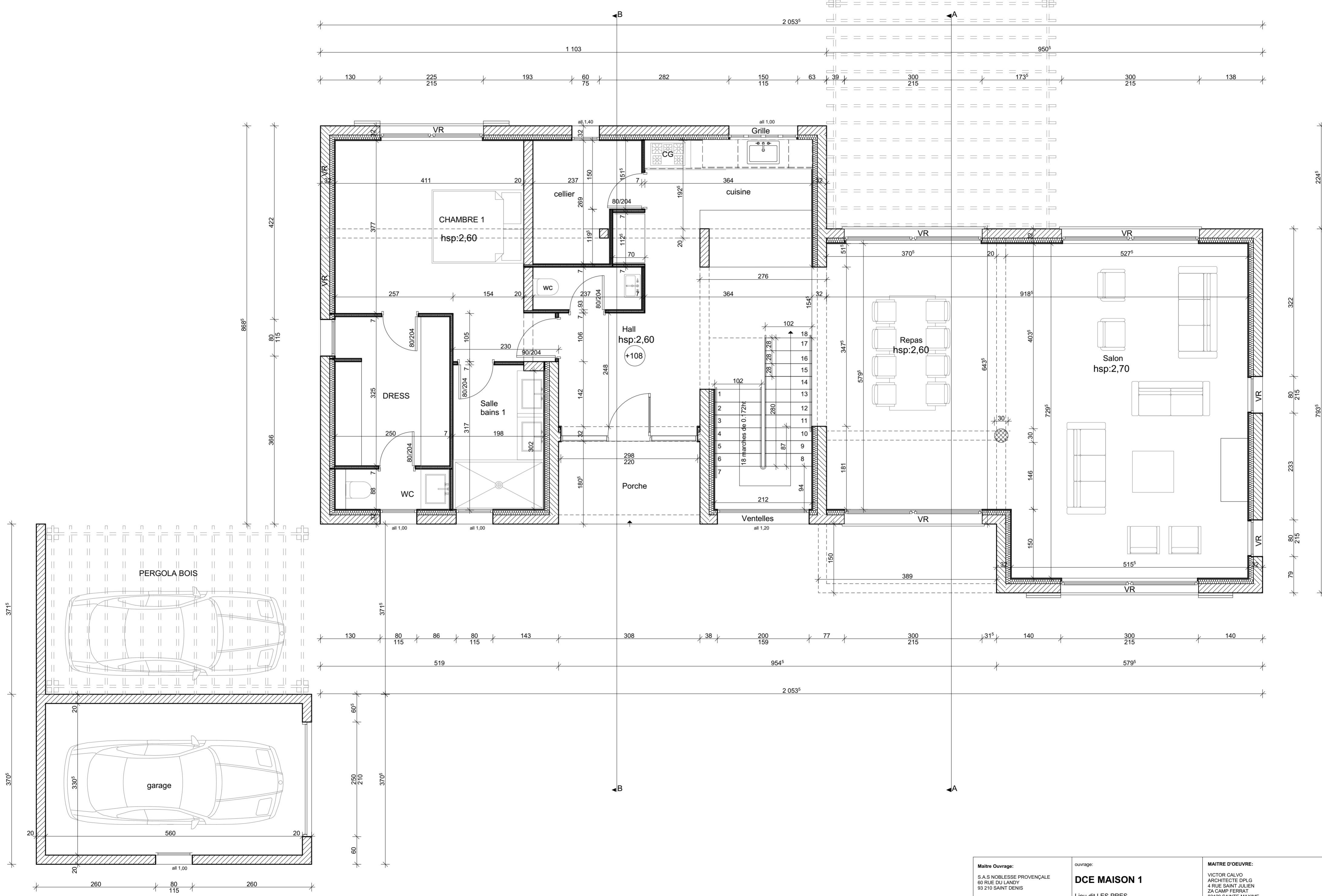
PLAN REZ DE CHAUSSEE
